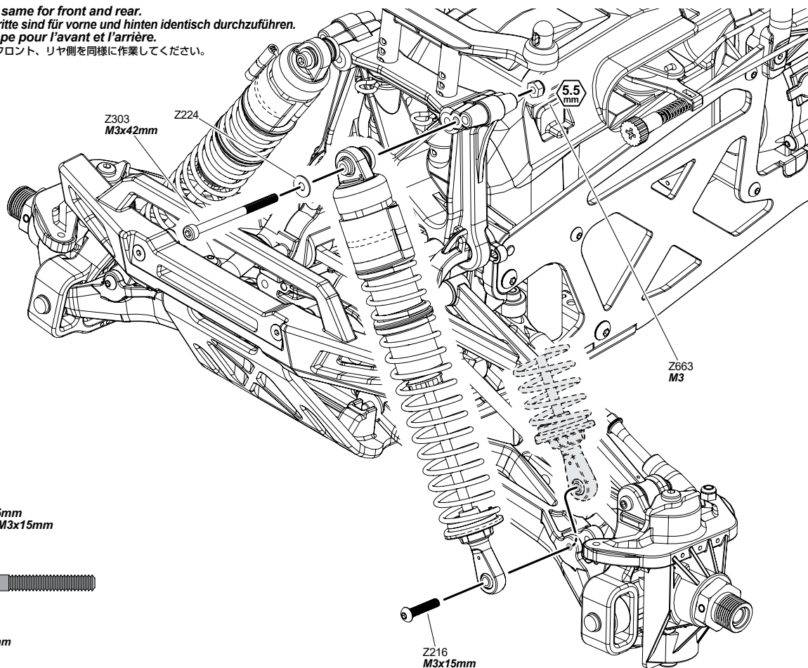
Allen Wrench Inbusschlüssel Clé Allen 六角レンチ 2.0mm / 2.5mm 2.0mm / 2.5mm 2.0mm / 2.5mm 2.0mm / 2.5mm
