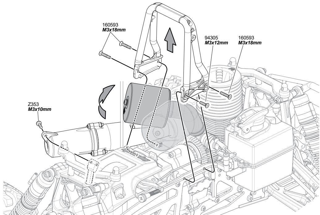
Allen Wrench 2.0mm / 3.0mm Inbusschlüssel 2.0mm / 3.0mm Clé Allen 2.0mm / 3.0mm 六角レンチ
