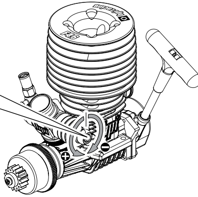
Flush (Factory Setting) Bündig (Werkseinstellung) En affleurement (réglage d'usine) キャブレター本体と同一面 (工場出荷初期設定)
