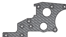
Carbon Rear Plate L (OPTIMA) カーボンリアプレートL (オブティマ)
