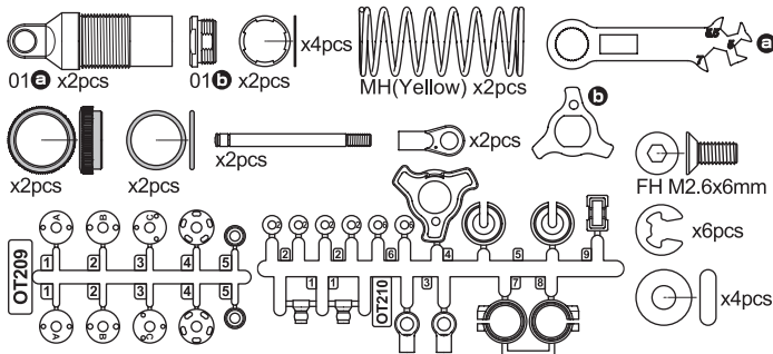
Gunmetal Front Damper (2pcs / OPTIMA MID) ガンメタルフロントダンパー (2入 / オプティマミッド)
