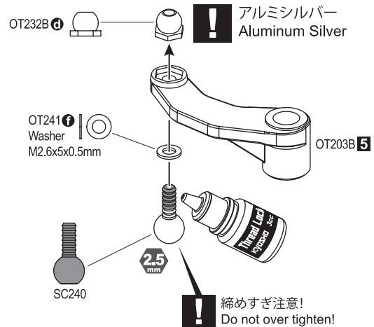
メタルサーボセイバー (オプティマ) Metal Servo Saver (OPTIMA)
