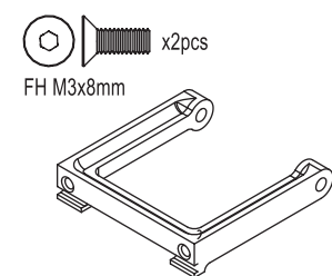
Hard Front Support (7075/OPTIMA) ハードフロントサポート (7075/オブティマ)
