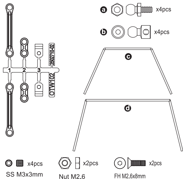
Stabilizer (OPTIMA) スタビライザー (オブティマ)
