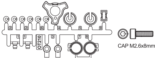
Shock Plastic Parts (Red/OPTIMA) ショックプラパーツ(レッド/オブティマ)
