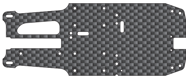
カーボンメカプレート (オブティマ) Carbon Radio Plate (OPTIMA)
