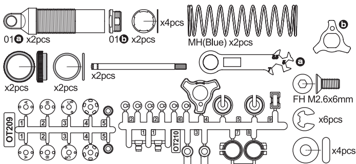
Gunmetal Rear Damper (2pcs / OPTIMA MID) ガンメタルリヤダンパー (2入 / オプティマミッド)
