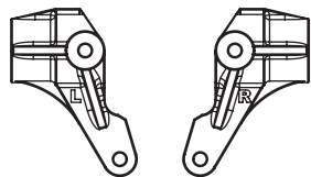
OT211B a x1 Knuckle Arm L ナックルアームL
