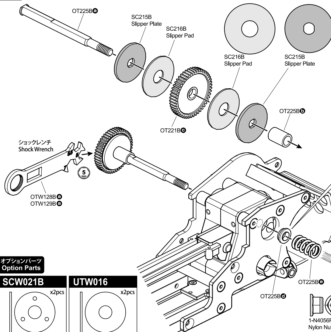
HD Slipper Pad (Scorpion 2014) HD スリッパパッド (2入/スコピオン2014)
