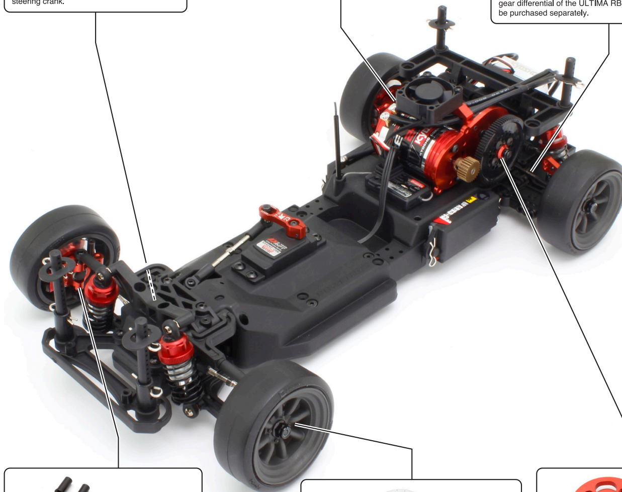
No.FAW303 ステアリングクラックピン(FZD2/2入) Steering Clank Pin (FZD2/2pcs) ステアリングクラックの剛性と精度を向上。 Improved rigidity and precision of the steering crank.
