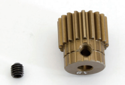
PNGA4819/4820/4822/ 4825/4832-37 ベルベットコートピニオンギヤ Velvet Coating Pinion Gear ※ (48P 19~22, 25, 32~37T)
