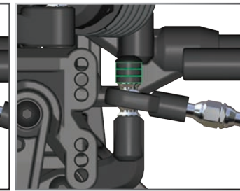
Ackerman máximo
