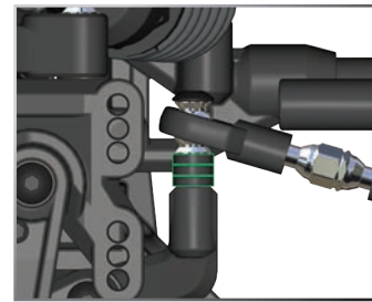
Ackerman mínimo
